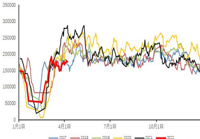
全国建筑钢材成交 (五日移动平均)
