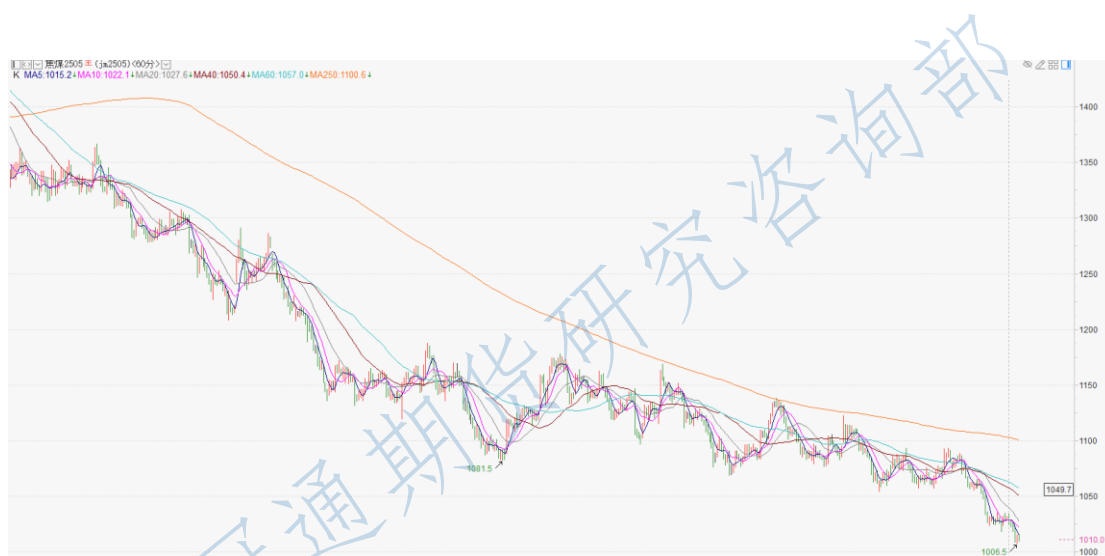
焦煤 2505 小时 K
