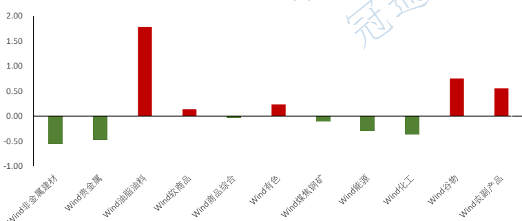
板块涨跌幅 (%)
